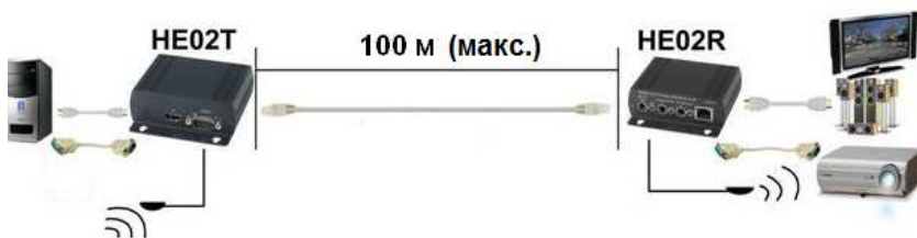
Рис. 3 Схема подключения HE02
