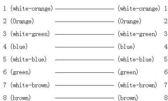
Прямой сетевой кабель
