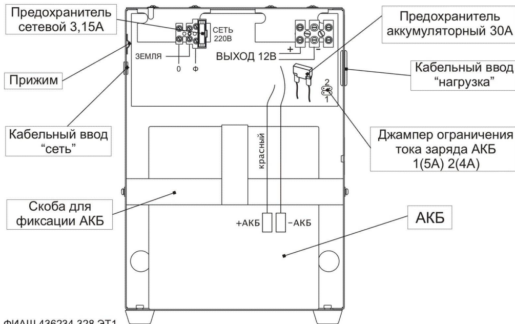
Рис.1 Расположение коммутационных элементов ВОЛНА ББП – 5/30 при снятой крышке корпуса
