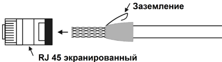
Рис.7 Соединение экранированного RJ 45 с кабелем STP
