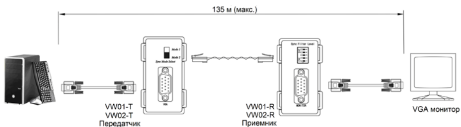
Рис.2 Структурная схема подключения VW01, VW02
