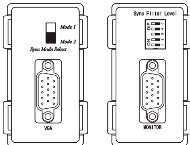
Рис.3 Разъемы и DIP-переключатели (VW01, VW02)
