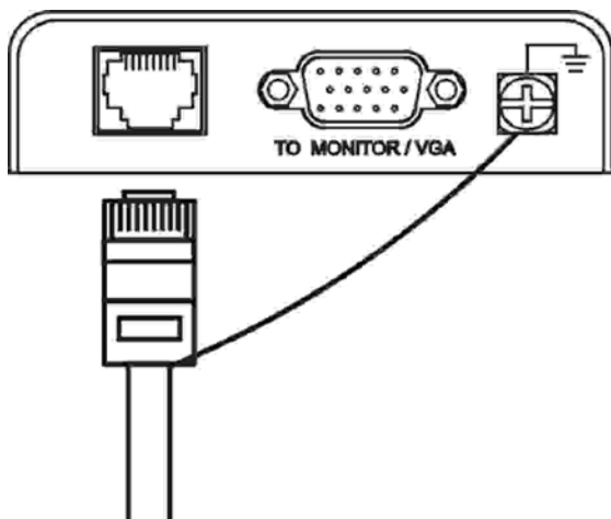
Рис. 9 Подключение кабеля заземления
