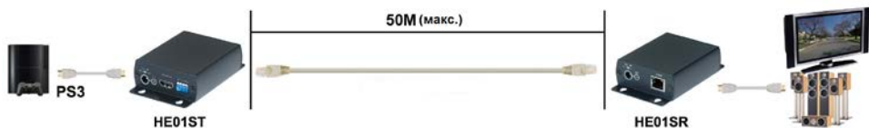
Рис. 9 Схема подключения передатчика HE01ST и приемника HE01SR.
