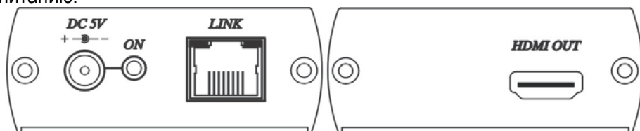
Рис.6 Панель подключения HE01SR
