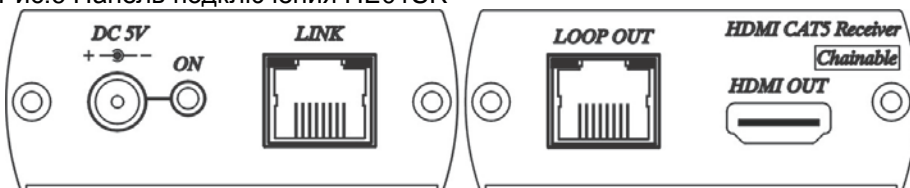
Рис.6 Панель подключения HE01SR
