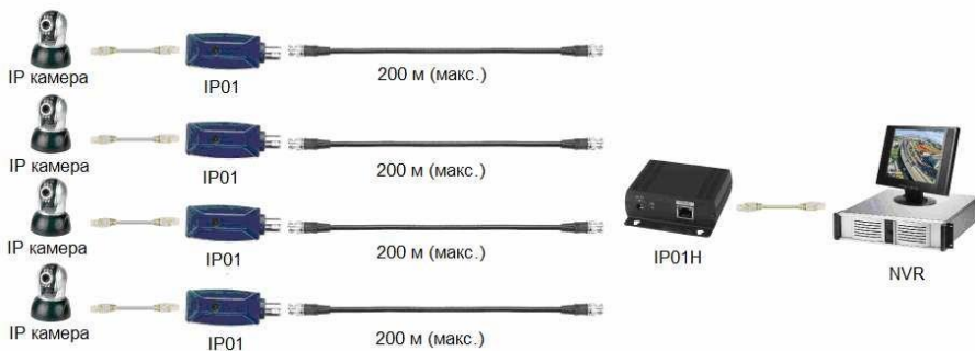
Рис. 3 Схема подключения
