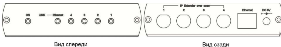
Рис. 4 Элементы IP01H
