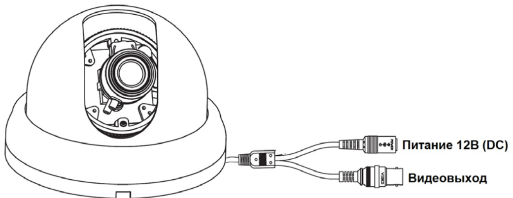
Рис.3.2.1. Подключение питания видеокamеры LTV-CDH-720-V2.8-12
