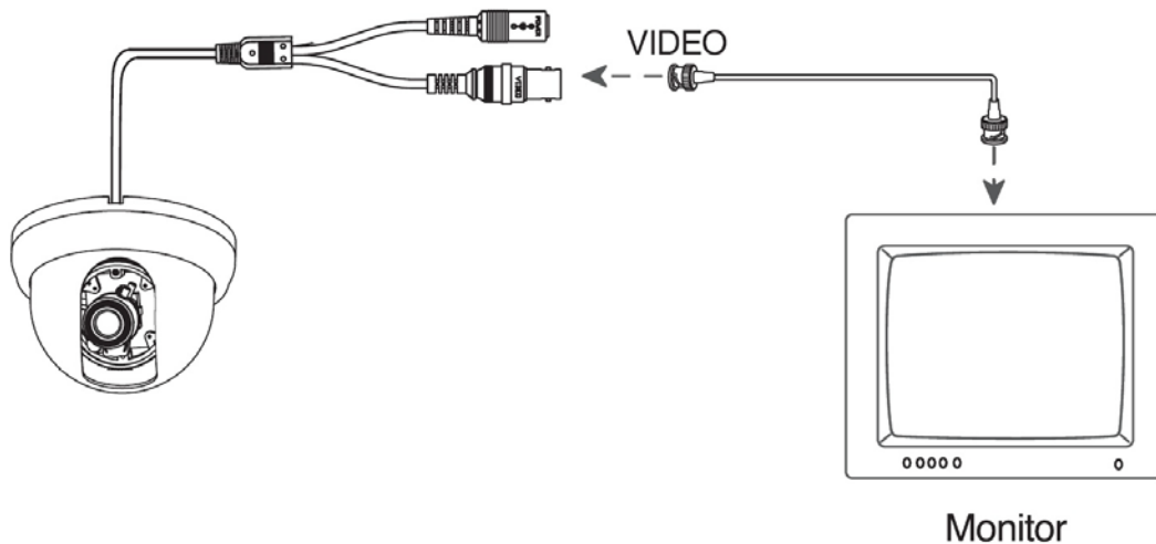
Рис.3.1.1. Подключение видеокамеры LTV-CDH-720(1)-V2.8-12 к монитору
