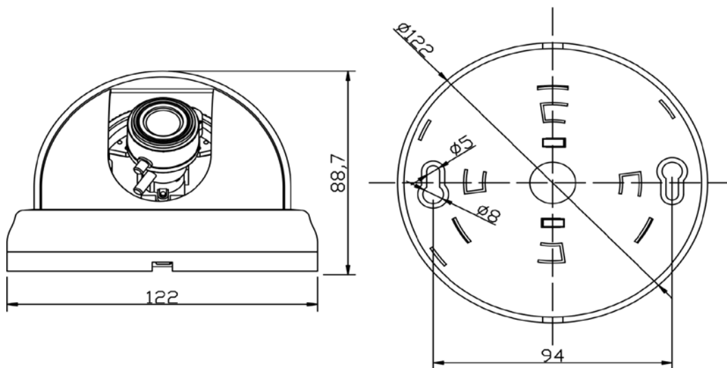
Рис.1.4.1. Габаритные размеры видеокамеры LTV-CDH-720(1)-V2.8-12
