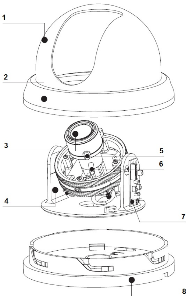
Рис.1.2.1. Основные компоненты видеокамеры LTV-CDH-720(1)-V2.8-12
