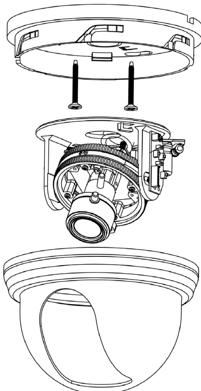
Рис.2.1.1. Установка видеокамеры LTV-CDH-720(1)-V на потолок/стену
