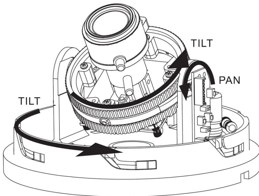
Рис.1.3.1. Настройка положения видеомодуля LTV-CDH-720(1)-V2.8-12
