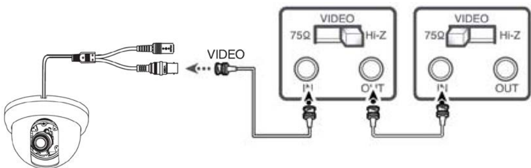
Рис.3.1.2. Подключение видеокамеры LTV-CDH-720(1)-V2.8-12 к монитору
