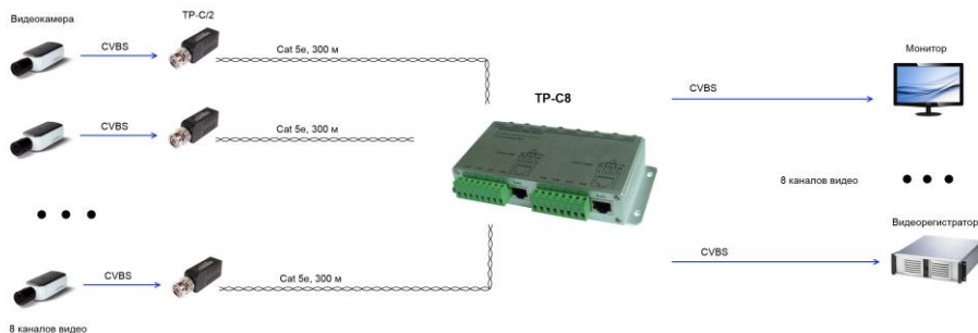
Рис.2 Схема подключения TP-C8
