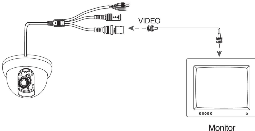
Рис.3.1.1. Подключение видеокамеры LTV-CDH-721W-V2.8-12 к монитору
