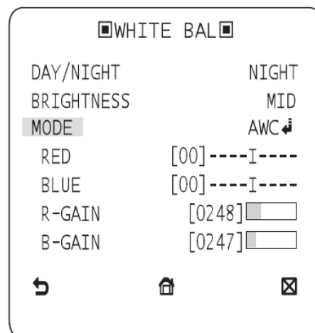
Рис.4.4.11.2. Подменю «WHITE BAL»
