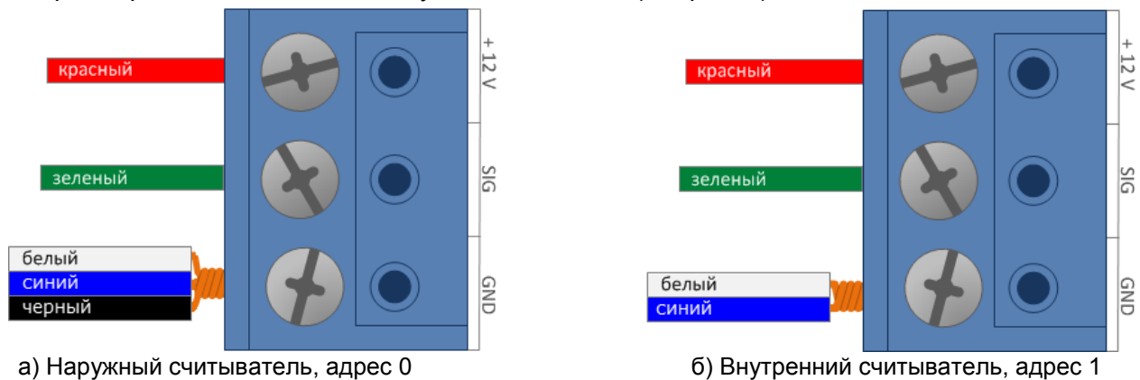
Рисунок 7. Подключение считывателя
