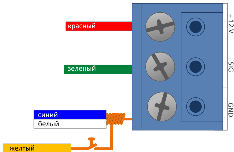
Рисунок 8. Пример подключения провода HOLD/SYNC для ручного включения режима блокировки
