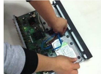
Падключыце SATA кабель і кабель харчавання на ніжняй і задняй частцы корпуса і зачыніце корпус верхняй вешкам.
