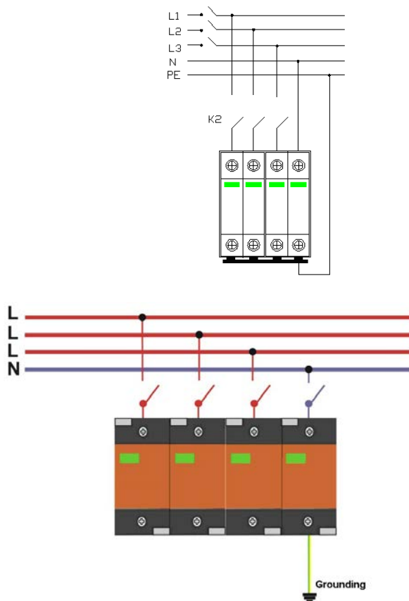
Рис.3 Подключение SP-AC3D/220-4, SP-AC3D/220-5
