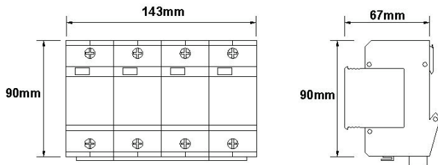
Рис.2 Габаритные размеры SP-AC3D/220-4, SP-AC3D/220-5
