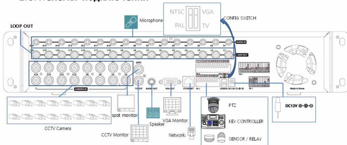
Рис. 2.1. Схема подключения оборудования к видеорегистратору SDRH-16M16
