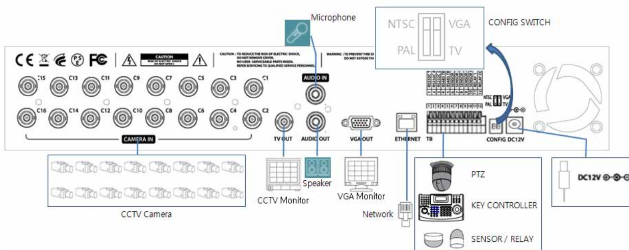
Рис. 2.2. Схема подключения оборудования к видеорегистратору SDRH-16E16
