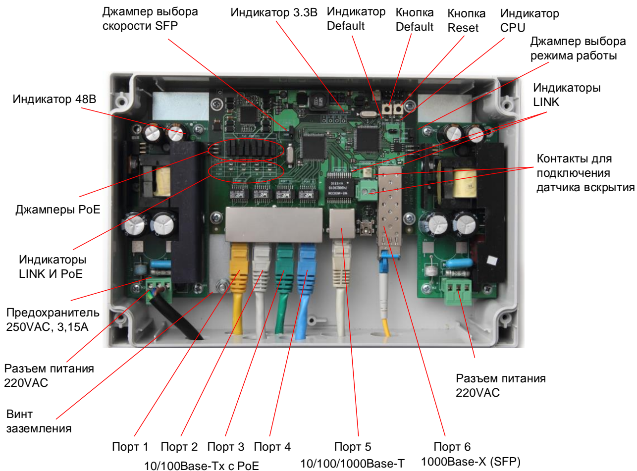
Рис. 2.2-1. Расположение элементов PSW -1G4F
