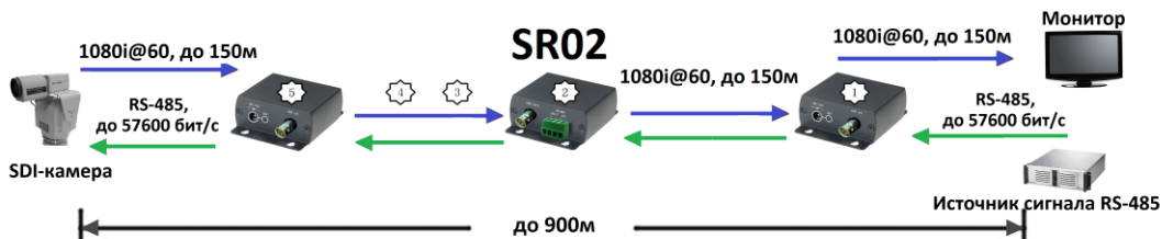
Рис. 5 Схема подключения каскадом SR02.
