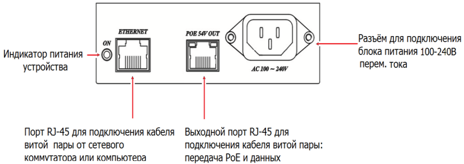
Рис.3 Разъёмы инжектора IP06I.
