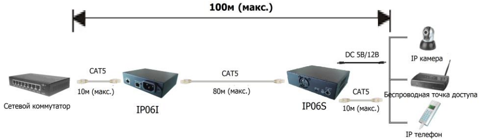
Рис.2 Схема подключения инжектора IP06I и сплиттера IP06S.
