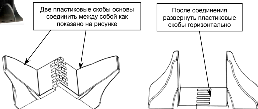
Рисунок 5. Сборка пластиковых основ для вертикальной установки источника
