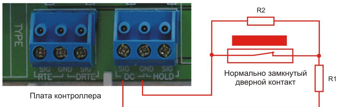
Рисунок 16. Подключение DC с контролем подводящих проводов
