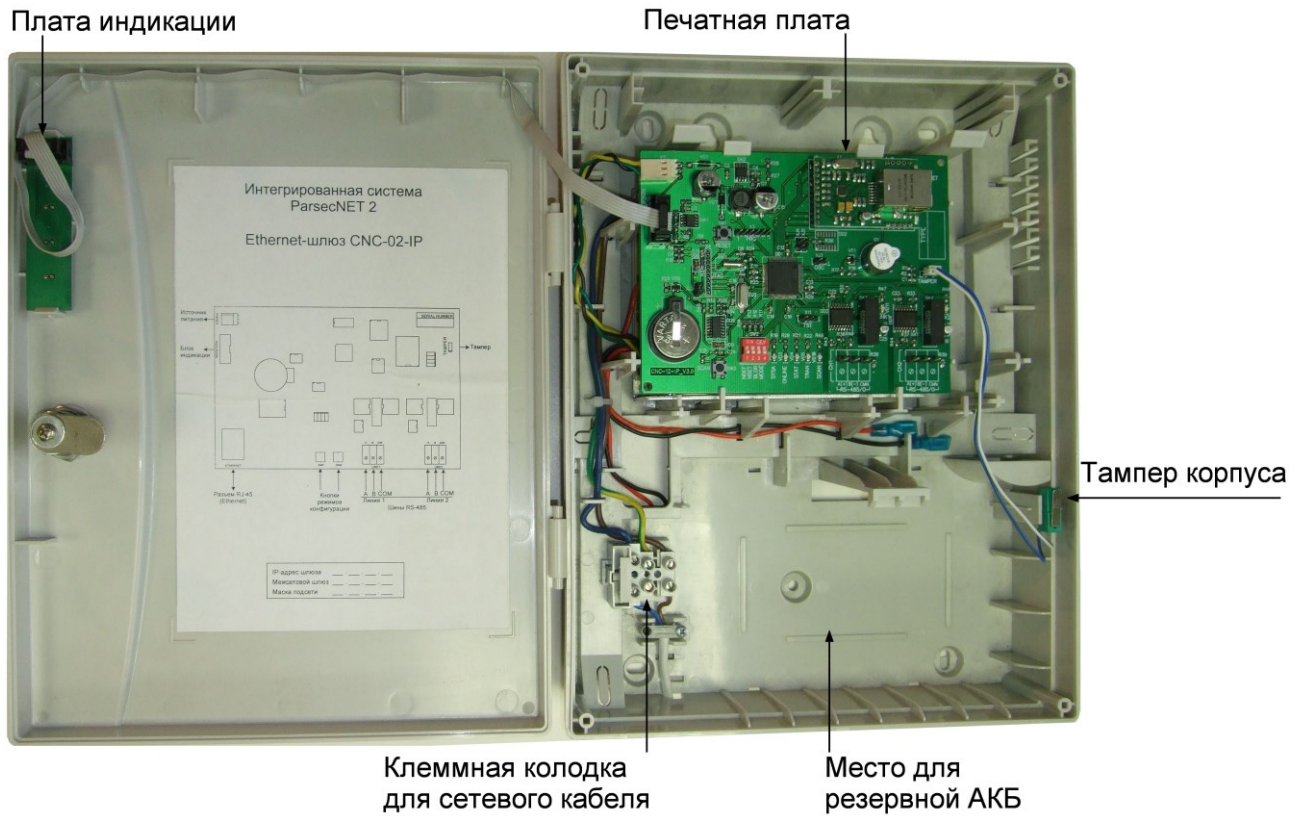
Рисунок 1. Открытый корпус шлюза
