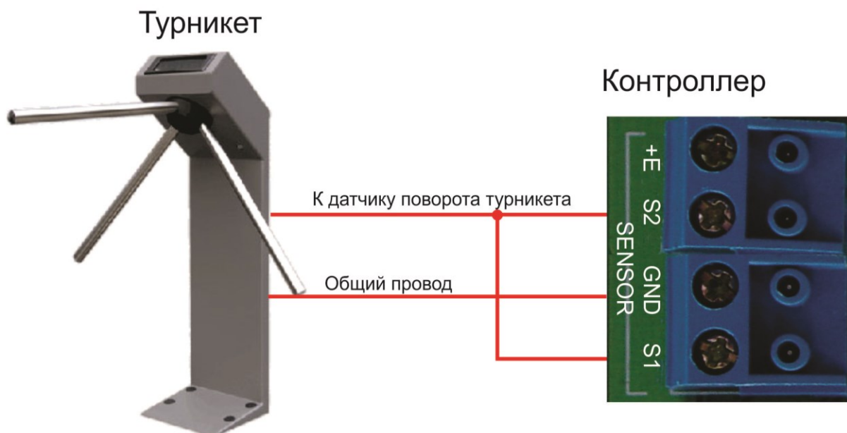
Рисунок 14. Подключение контроллера к турникету с одним датчиком поворота
