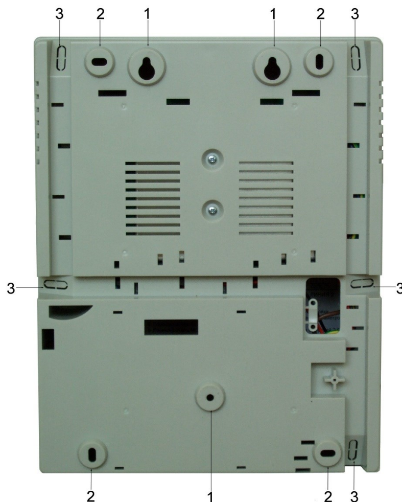
Рисунок 4. Монтажные отверстия
