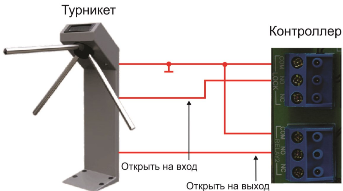
Рисунок 13. Управление турникетом контроллером
