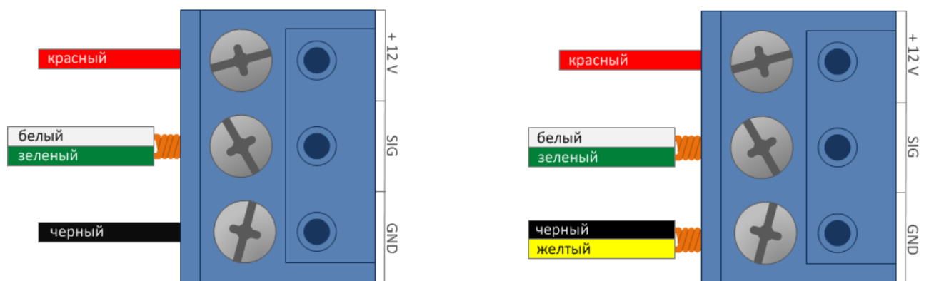
Рисунок 3. Подключение считывателя в режиме Parsec
