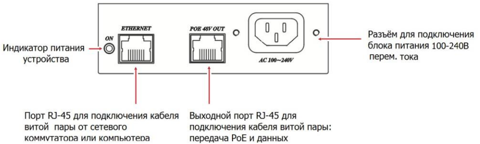
Рис.3 Разъёмы инжектора IP051.
