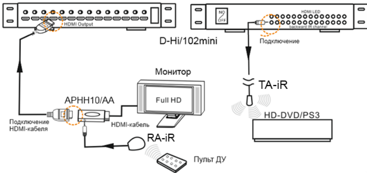
Рис. 4 Схема работы с ИК-сигналом
