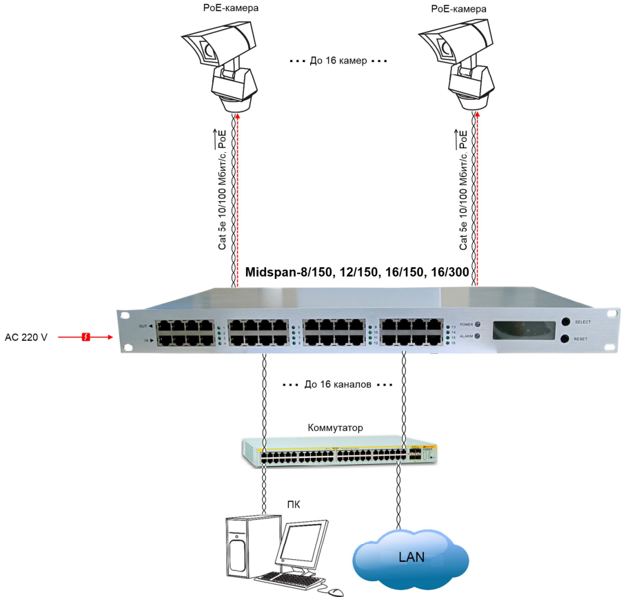
Рис. 3 Схема подключения PoE Инжекторов
