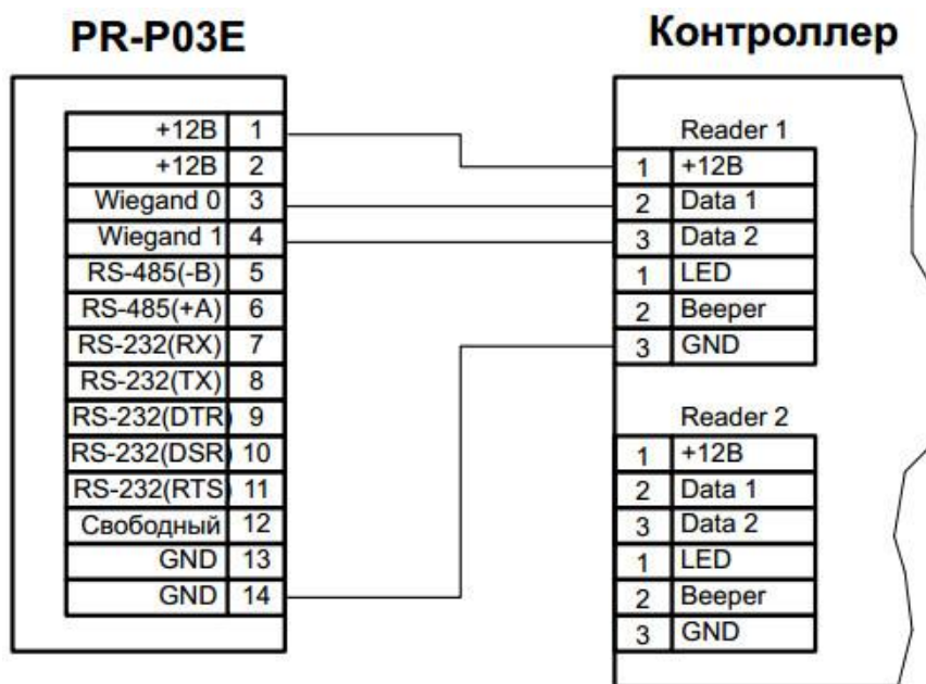
Рисунок 1. Схема подключения
