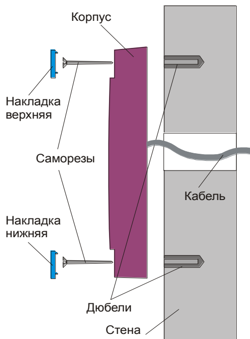
Рисунок 2. Крепление считывателя
