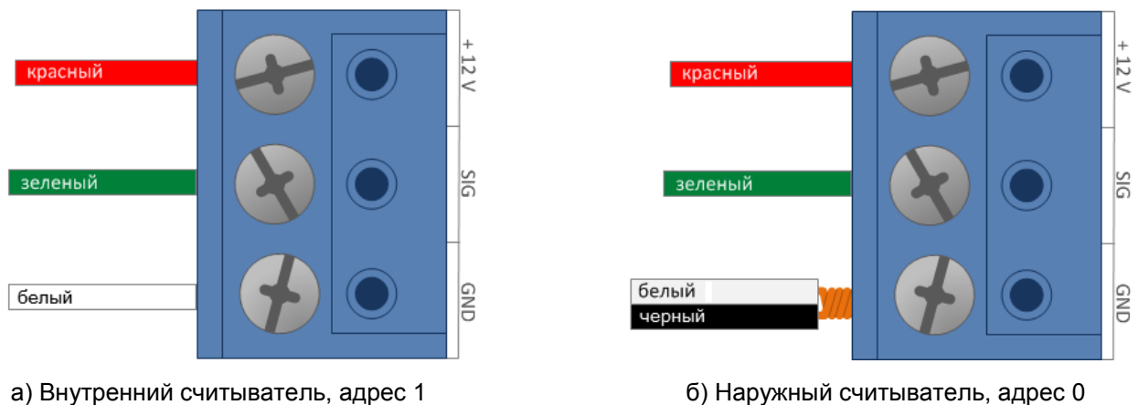
Рисунок 8. Подключение счетчика в режиме «карта + ПИН»
