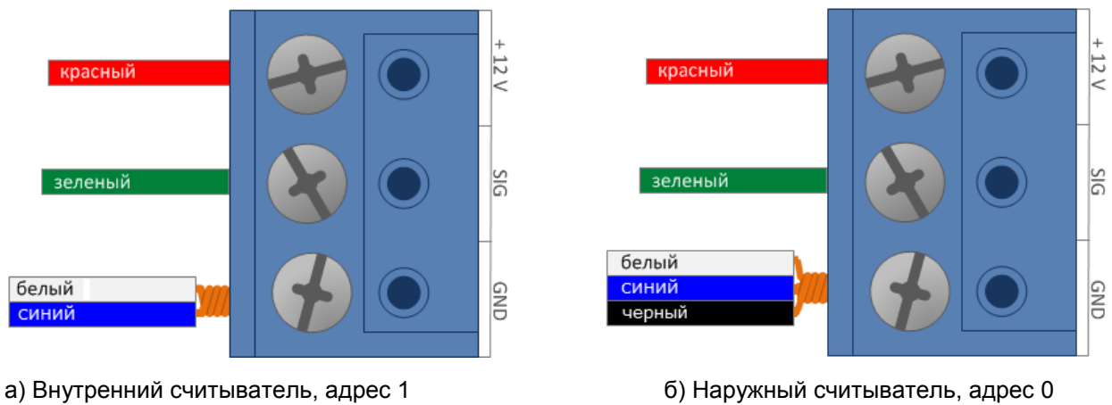
Рисунок 7. Подключение счетчика в режиме «только карта»
