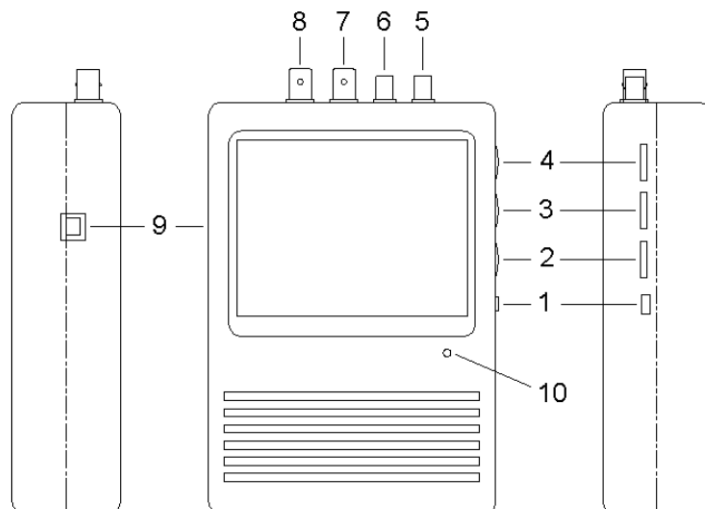
Рис.2.1. Строение и функции LTV-MCL-43T
