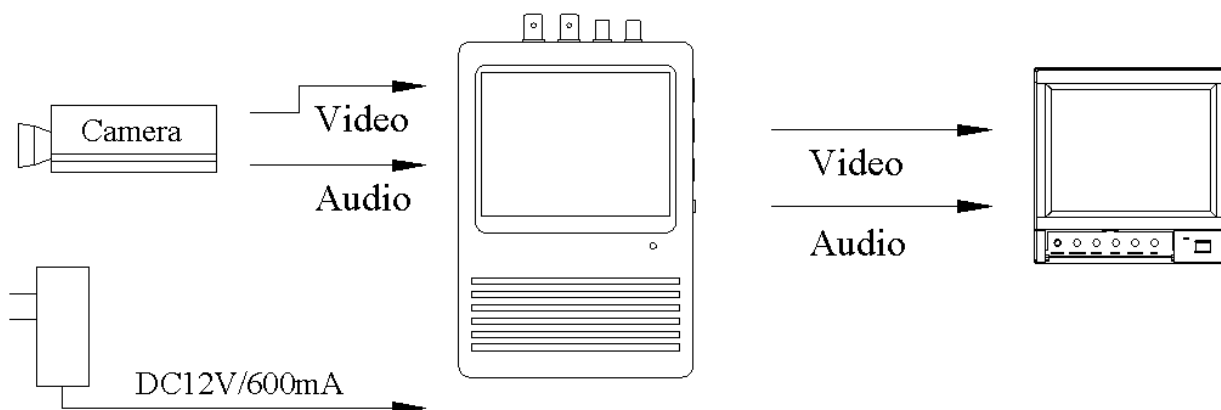
Рис.4.1. Схема подключения LTV-MCL-43T
