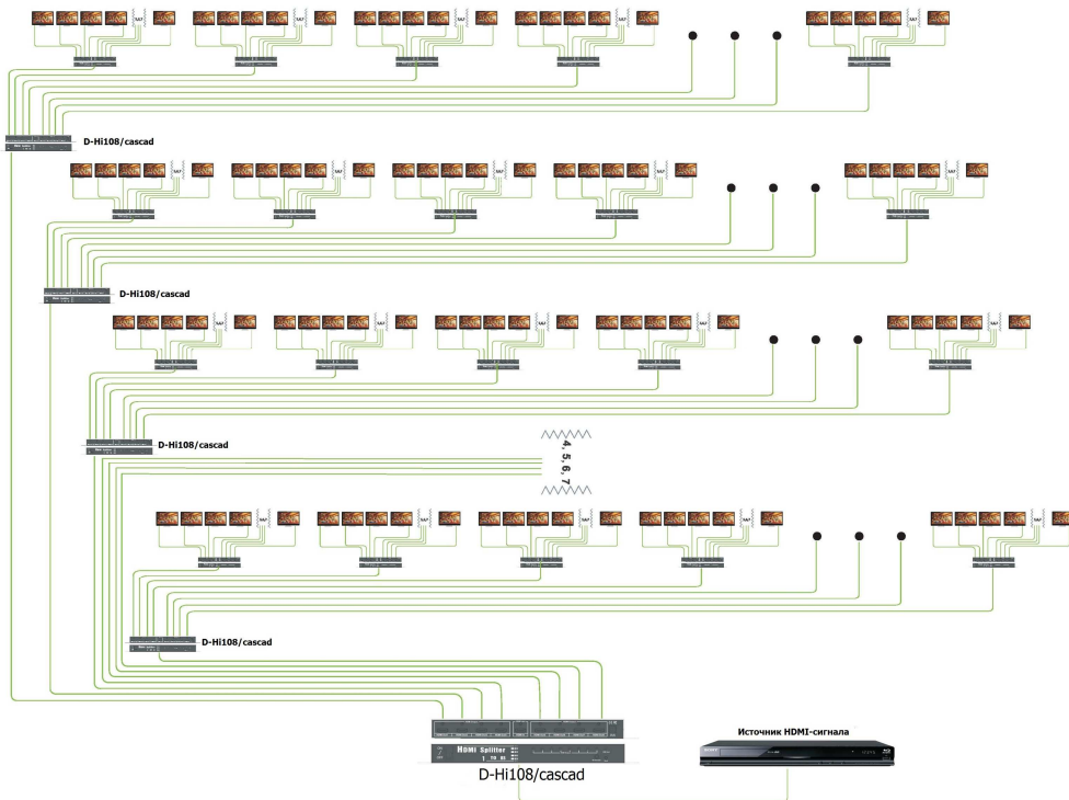
Рис. 3 Схема подключения разветвителя D-Hi108/cascad
